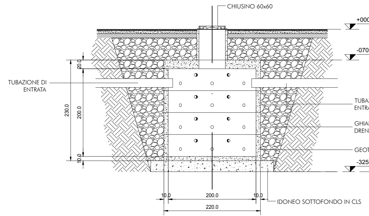
SCALA 1:50 PARTICOLARE POZZO PENDENTE
